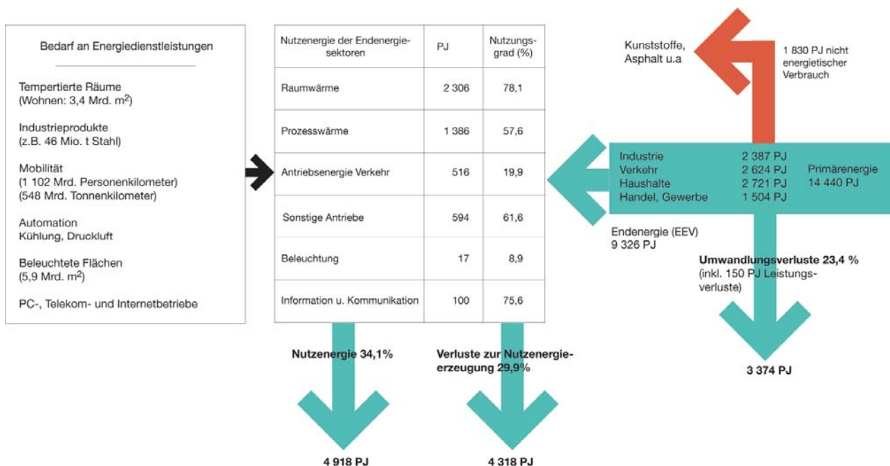
Abbildung 4-1: Energieflussdiagramm und Energieverluste auf allen drei Stufen der Energienutzung und -wandlung, Deutschland 2004. Quelle: Fraunhofer-ISI (2006)
